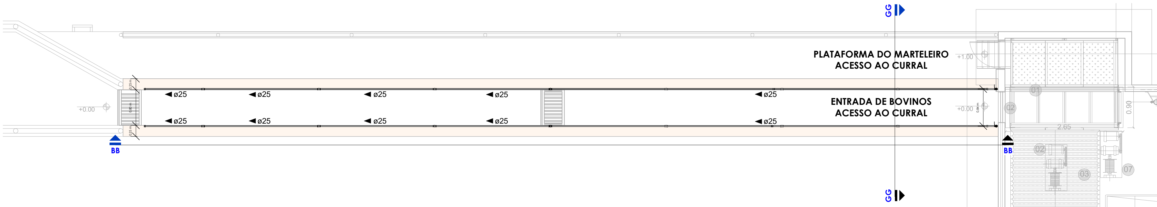
PLANTA BAIXA _ SERINGA_BOVINOS - ESC
