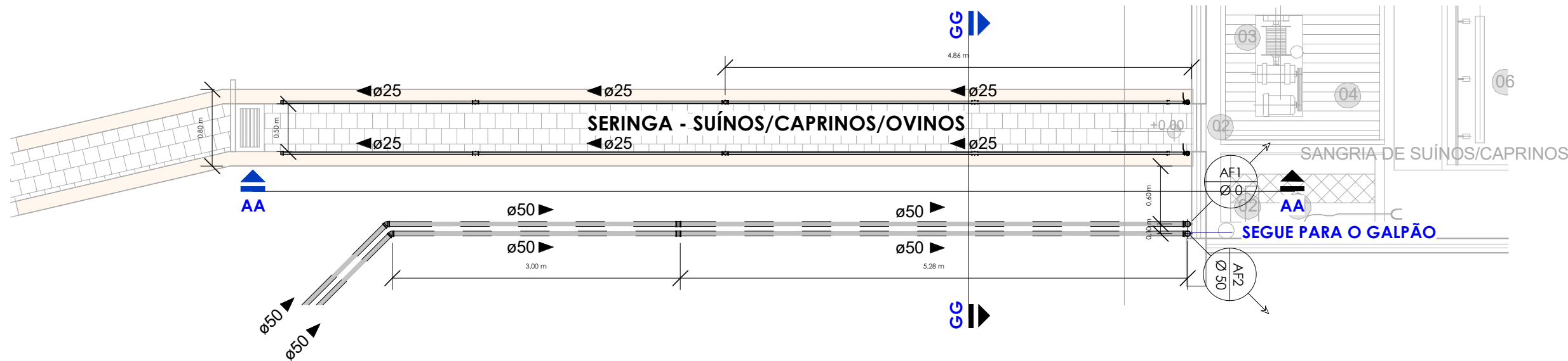
PLANTA BAIXA _ SERINGA - SUÍNOS/CAPRINOS/OVINOS - ESC
